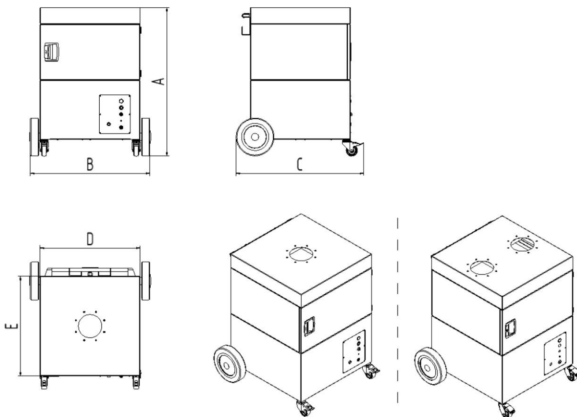
Bild 18: Måttblad 60650 + 60650DA
