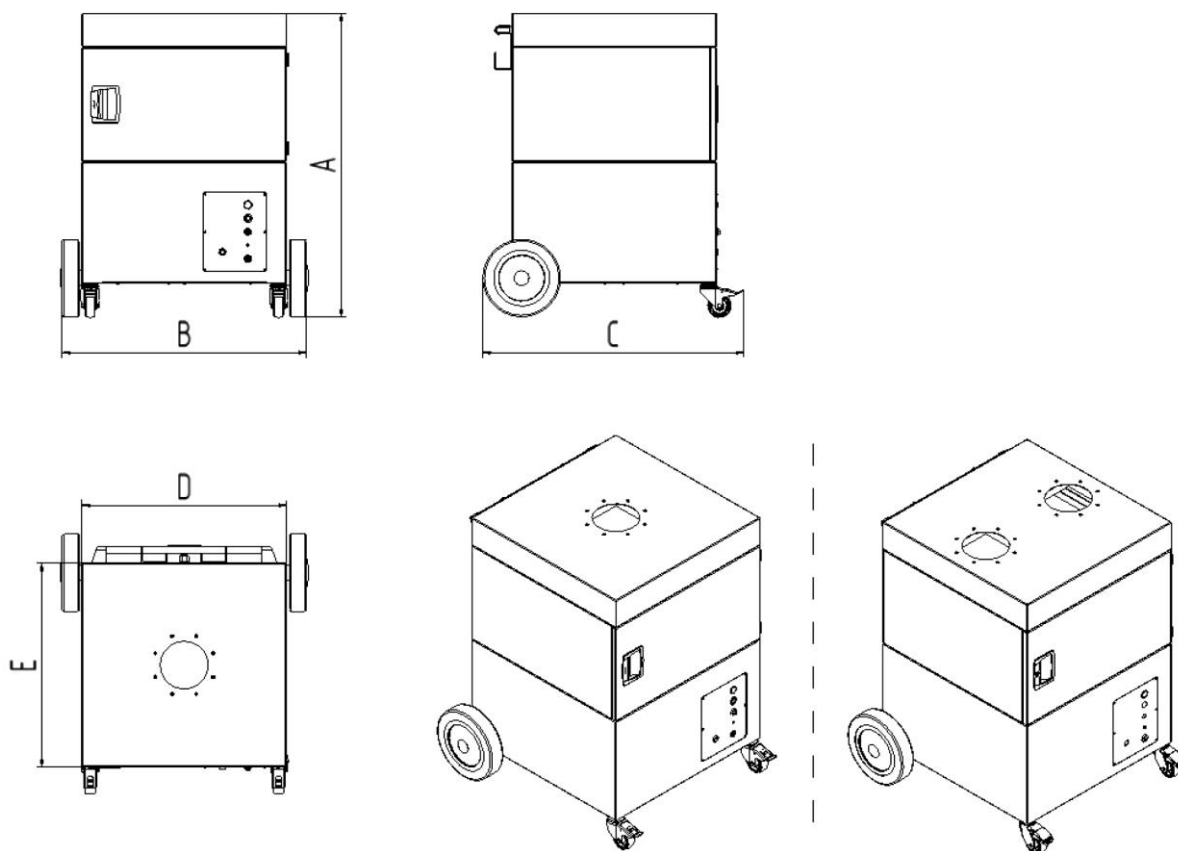
Kuva 27: Mittalehti 60650 + 60650DA
