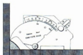
Fillet Leg Length
